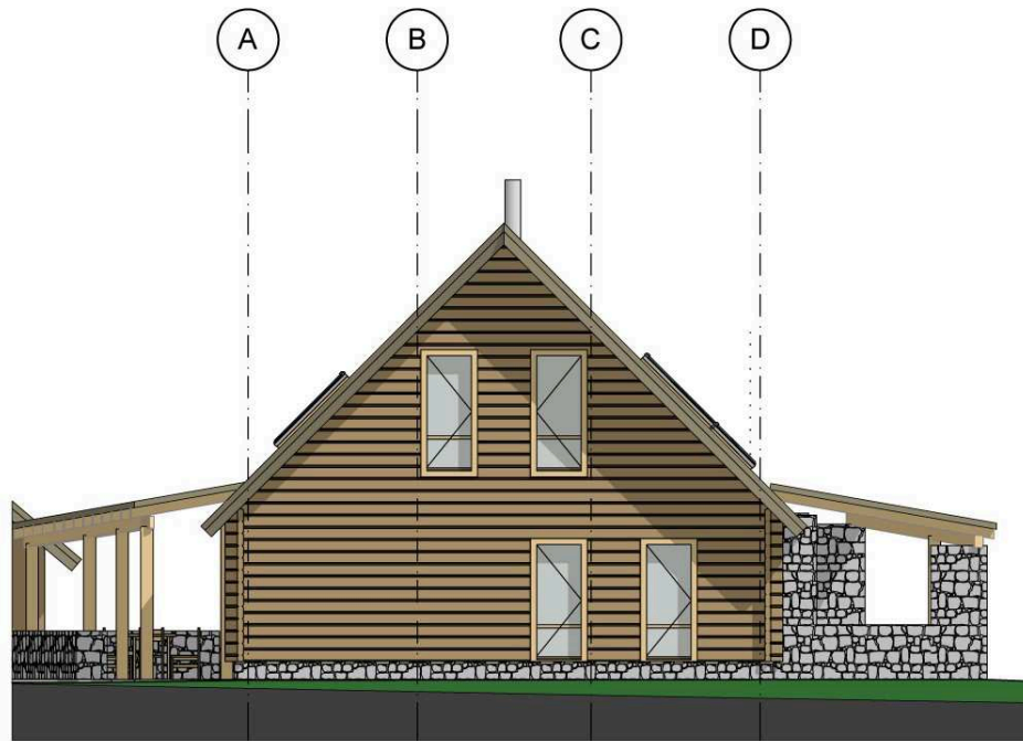
E2 Elewacja zachodnia 1:100
