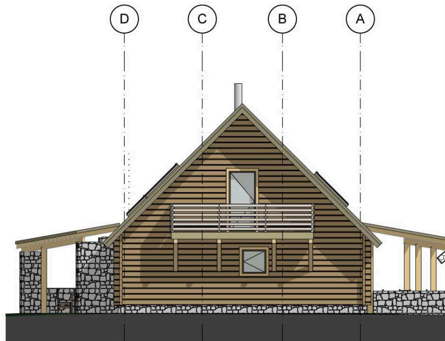
E4 Elewacja wschodnia 1:100
